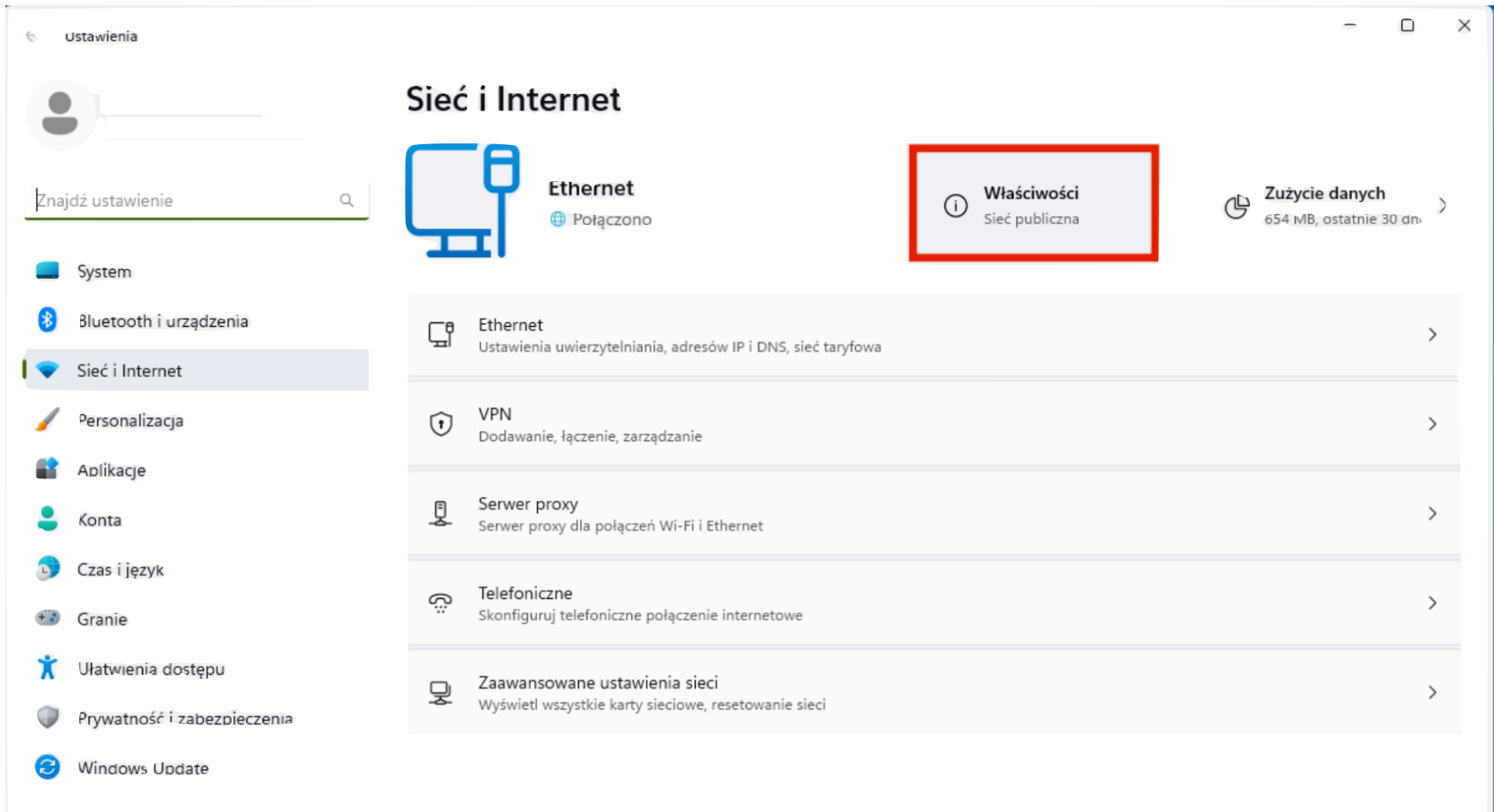
Rys. 3. Wciśnij "Właściwości"
